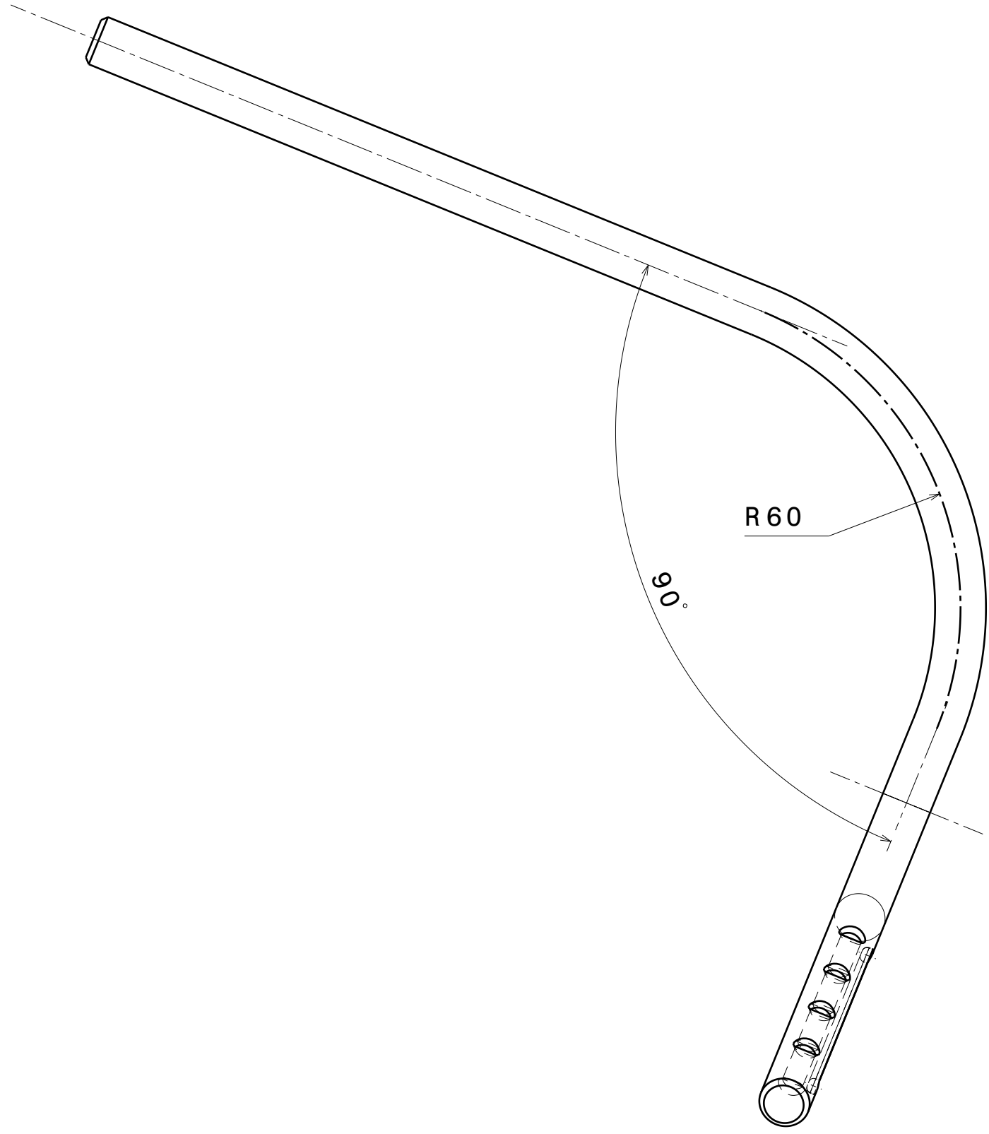
VISTA AUXILIAR E ESCALA: 1:1
